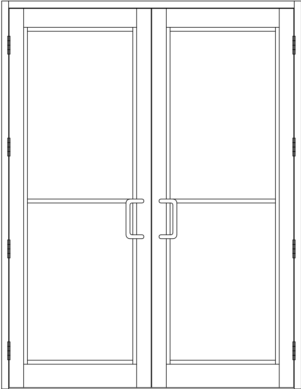
SE 3550 STOREFRONT (LARGE MISSILE IMPACT)
